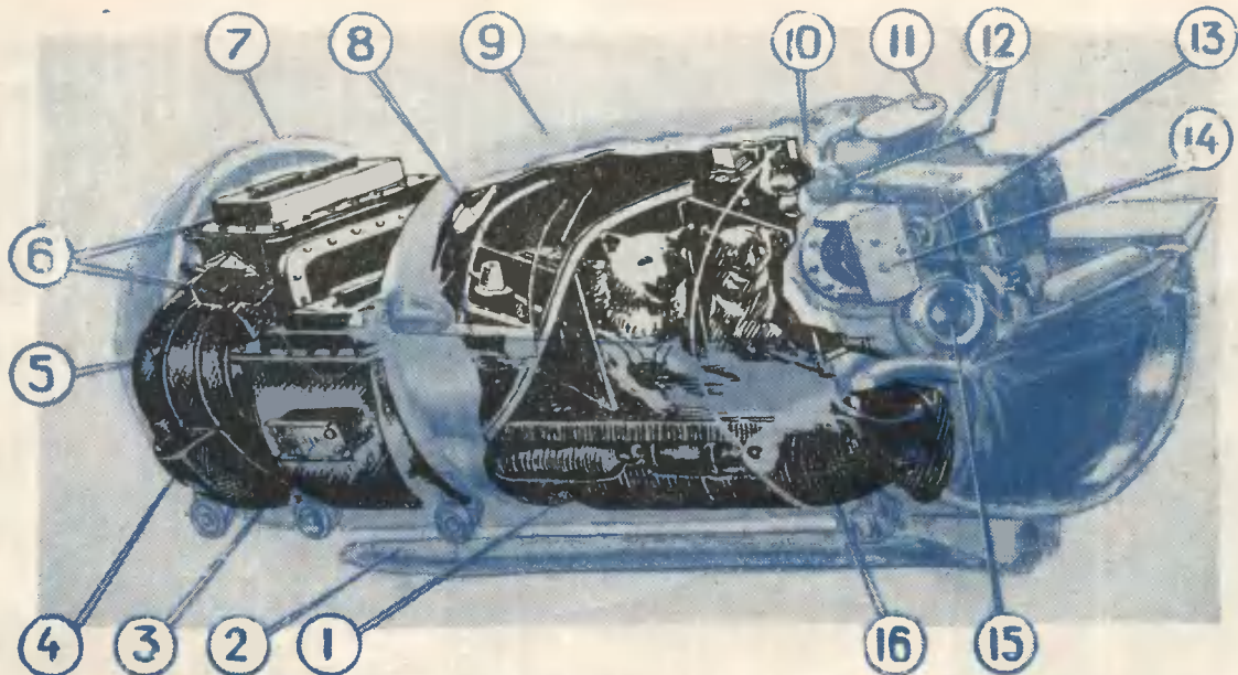
ГЕРМЕТИЧЕСКАЯ КАБИНА ЖИВОТНЫХ В КАТАПУЛЬТИРУЕМОМ КОНТЕЙНЕРЕ НА БОРТУ КОРАБЛЯ-СПУТНИКА
